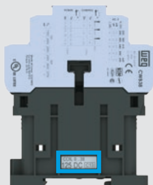
Bobina CC
